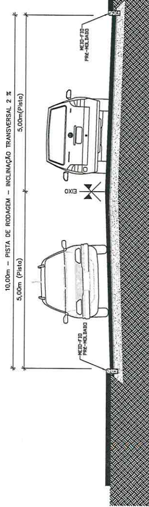
SEÇÃO TIPO DE PAVIMENTAÇÃO ASFÁLTICA - LOTEAMENTO COSTA SUL
